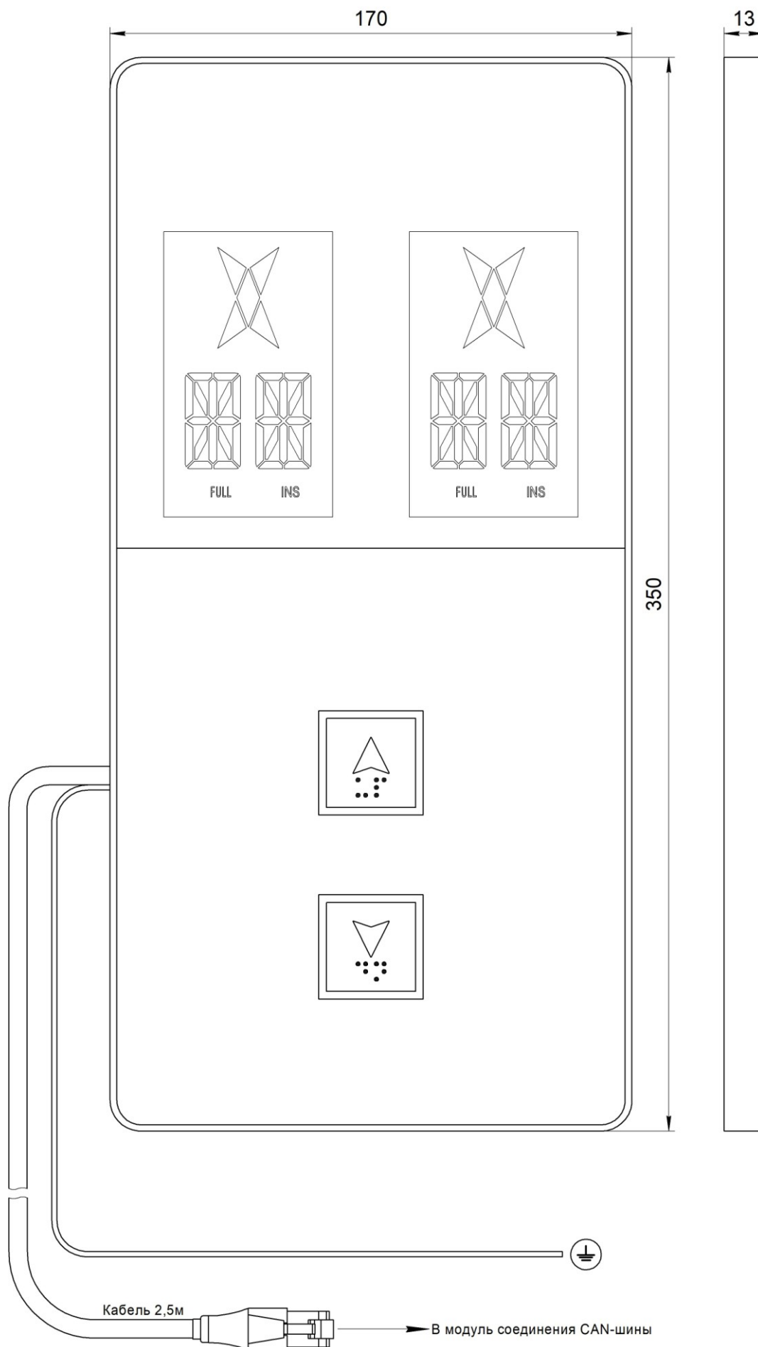
Рис.1 Внешний вид, габаритные и установочные размеры Вызывного поста МАЛАХИТ (жгут RJ45) НШЕК.468381.112
